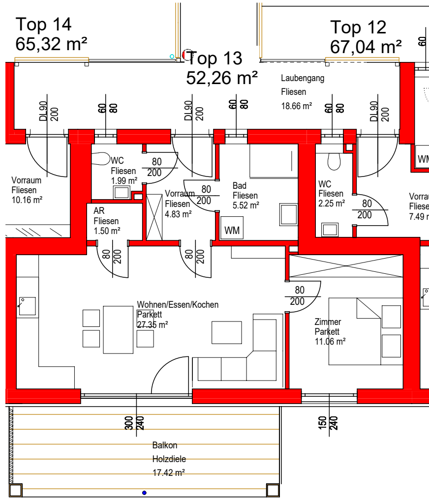
2. Obergeschoss
