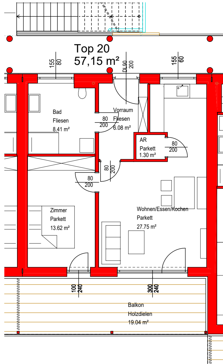
1. Obergeschoss
