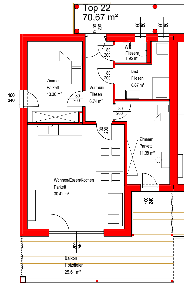
1.Obergeschoss
