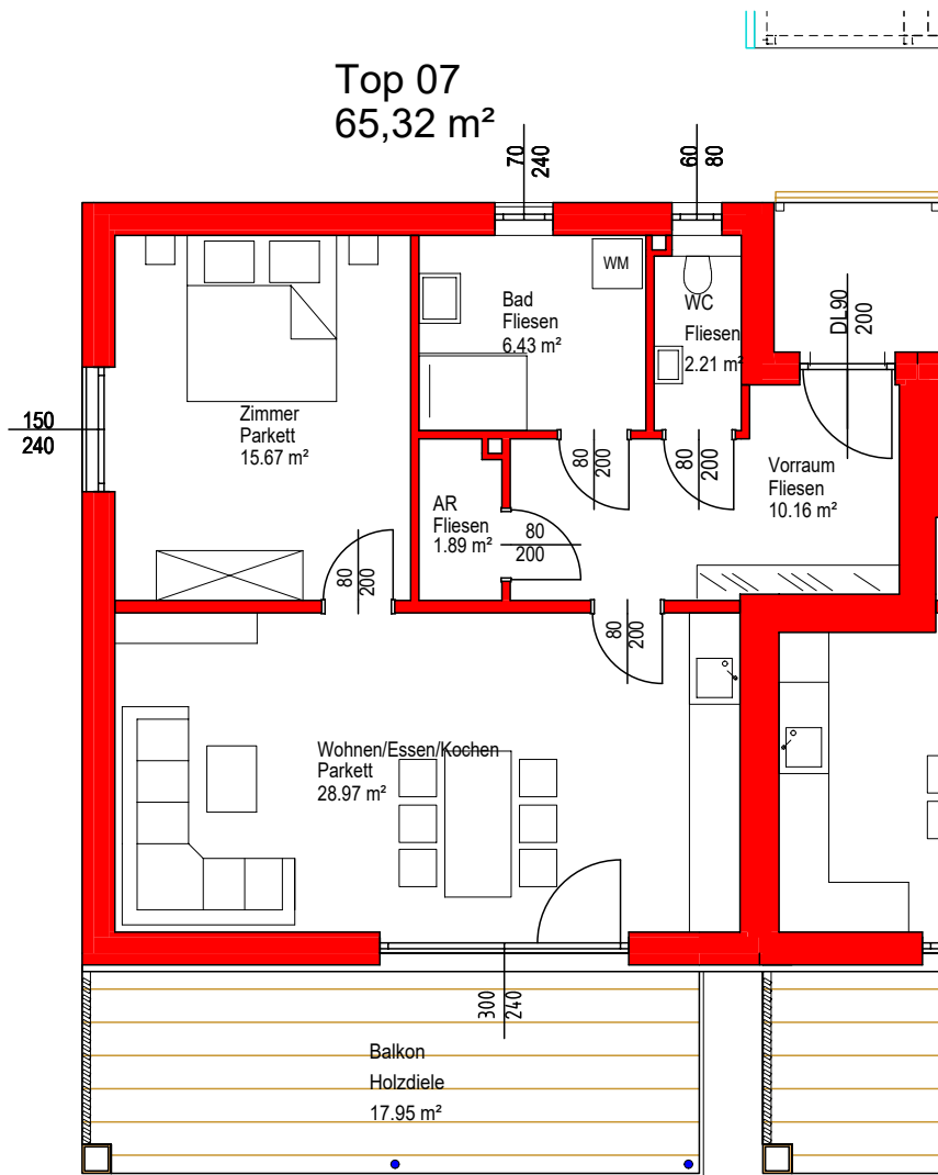
2.Obergeschoss
