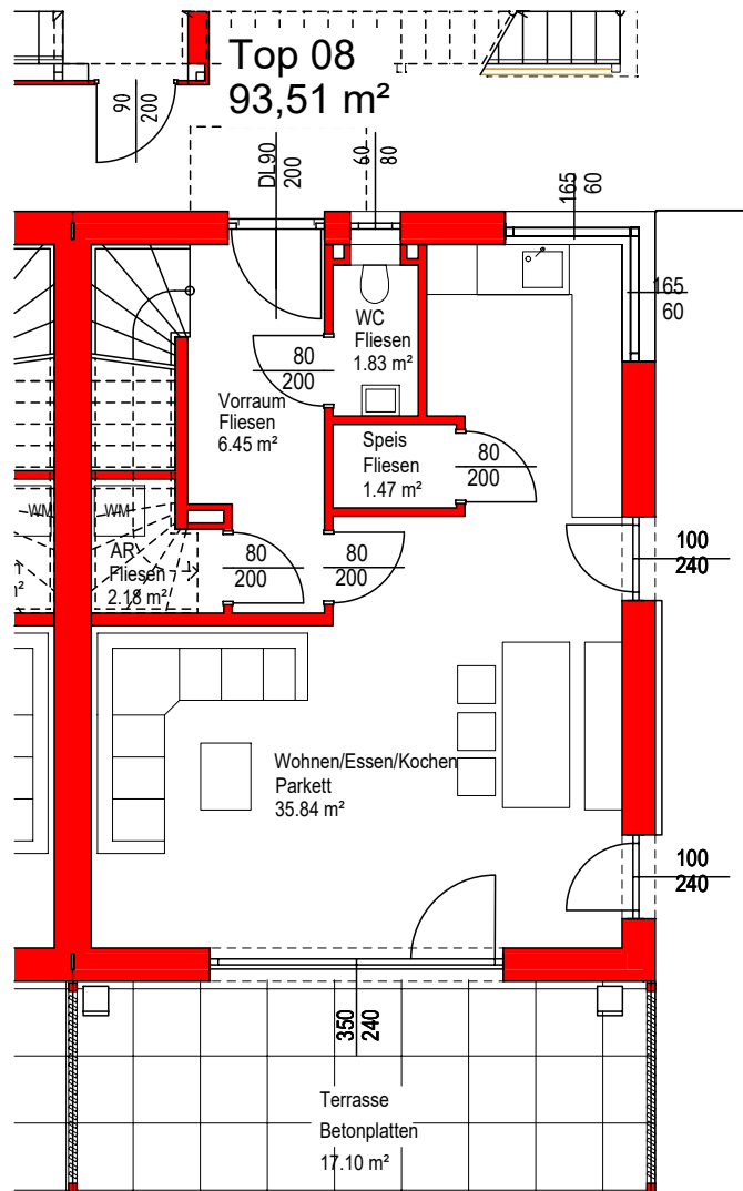
Erdgeschoss
