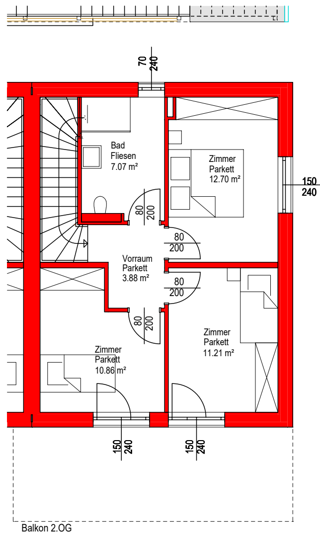
Obergeschoss
